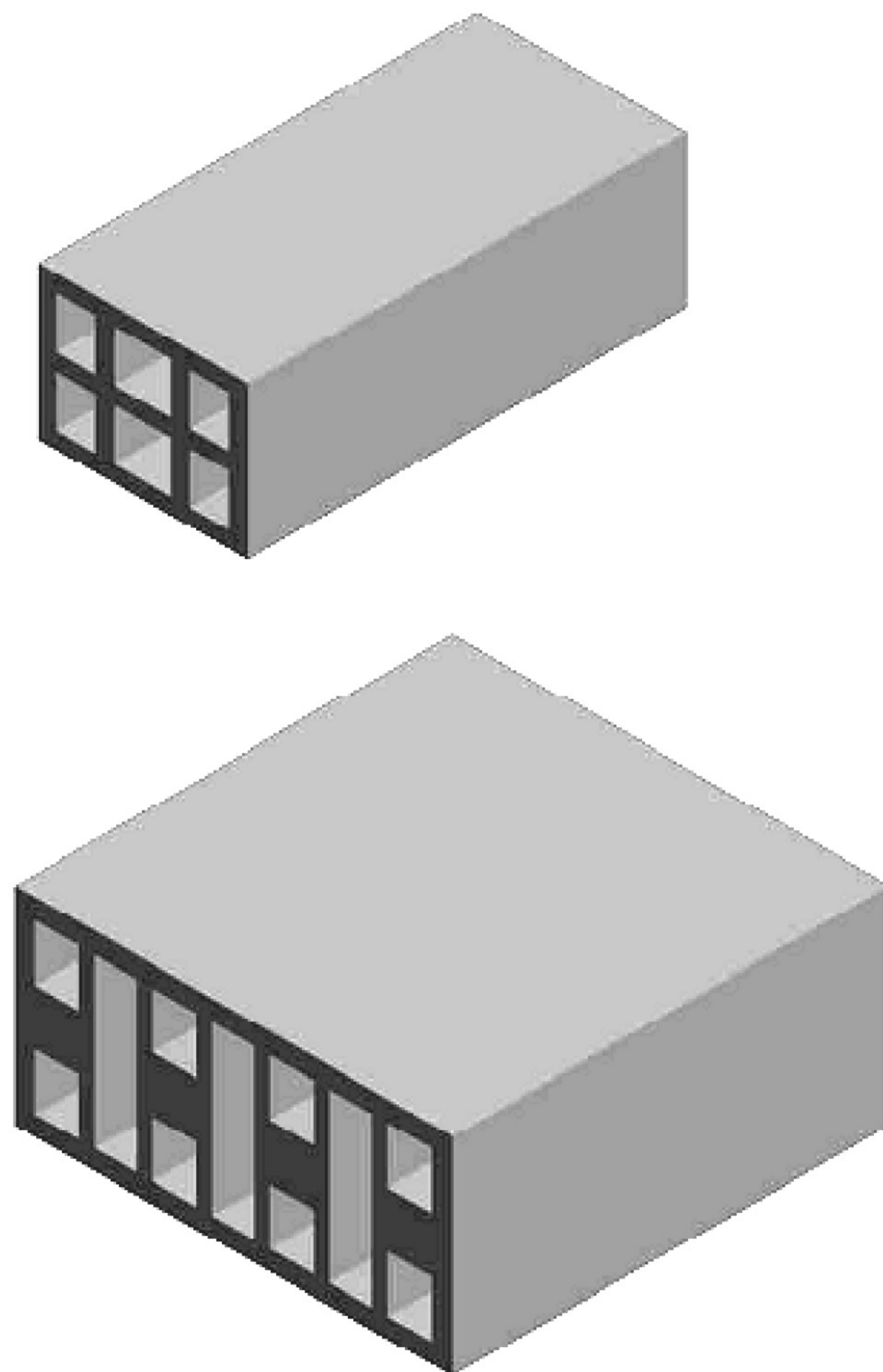
Рисунок А.2 — Изделия с горизонтальными пустотами
