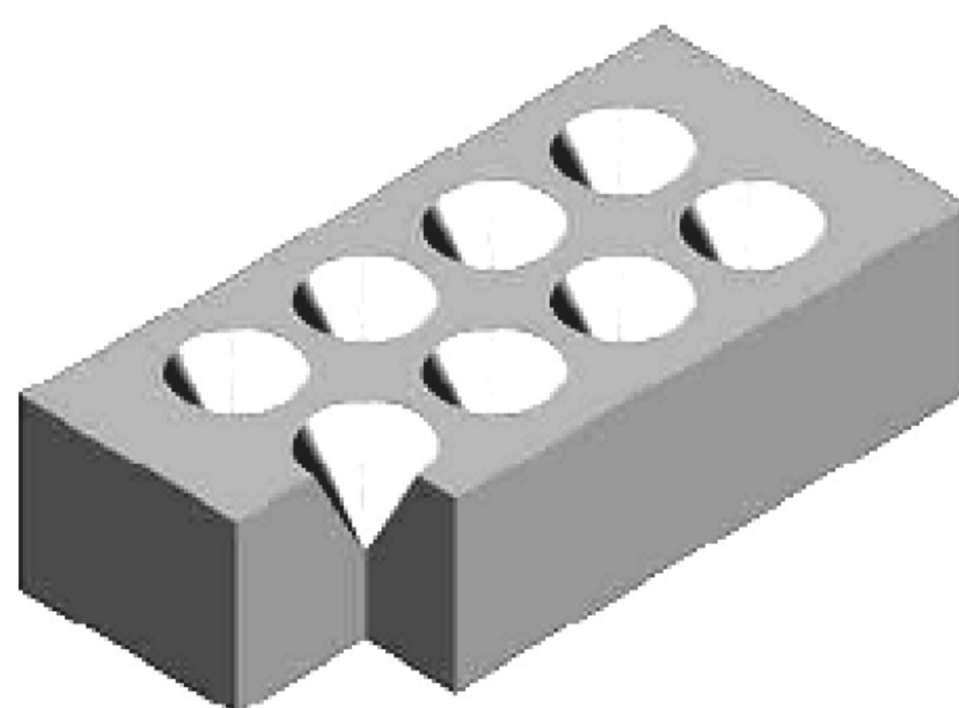
Рисунок А.3 — Изделие с несквозными пустотами
