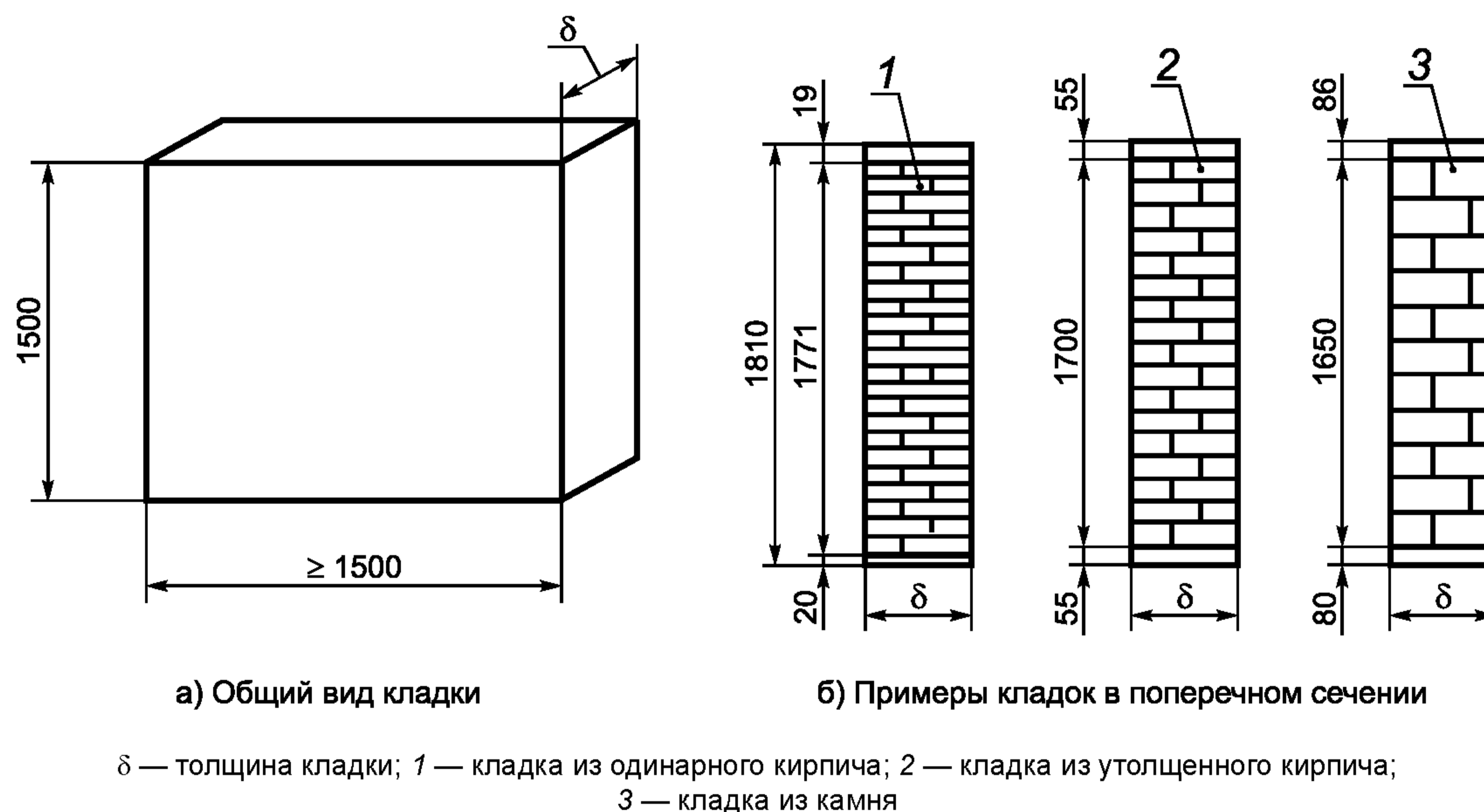
Рисунок 2 — Фрагмент кладки для определения коэффициента теплопроводности
