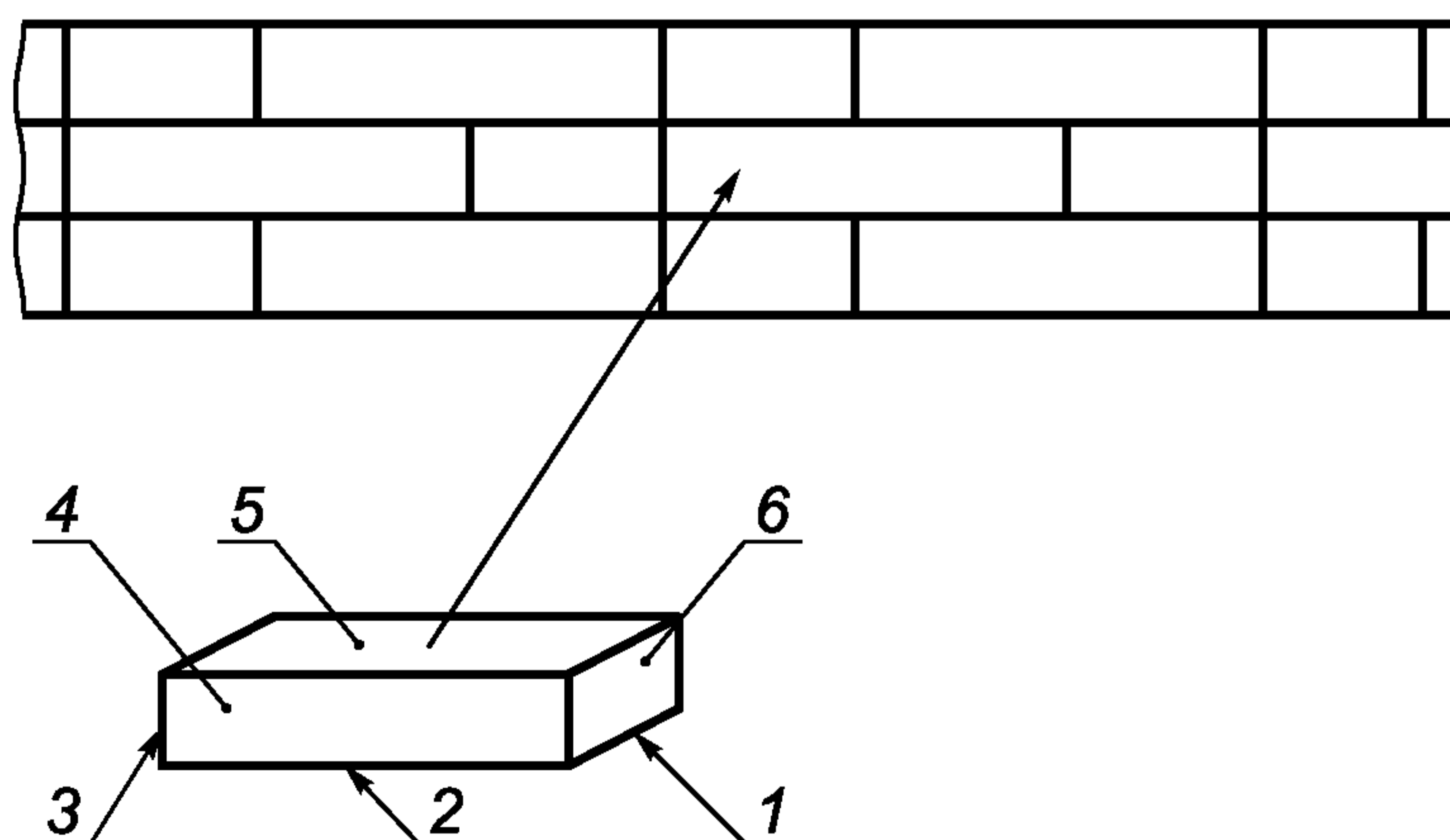
1 — ширина; 2 — длина; 3 — толщина; 4 — ложок; 5 — постель; 6 — тычок
