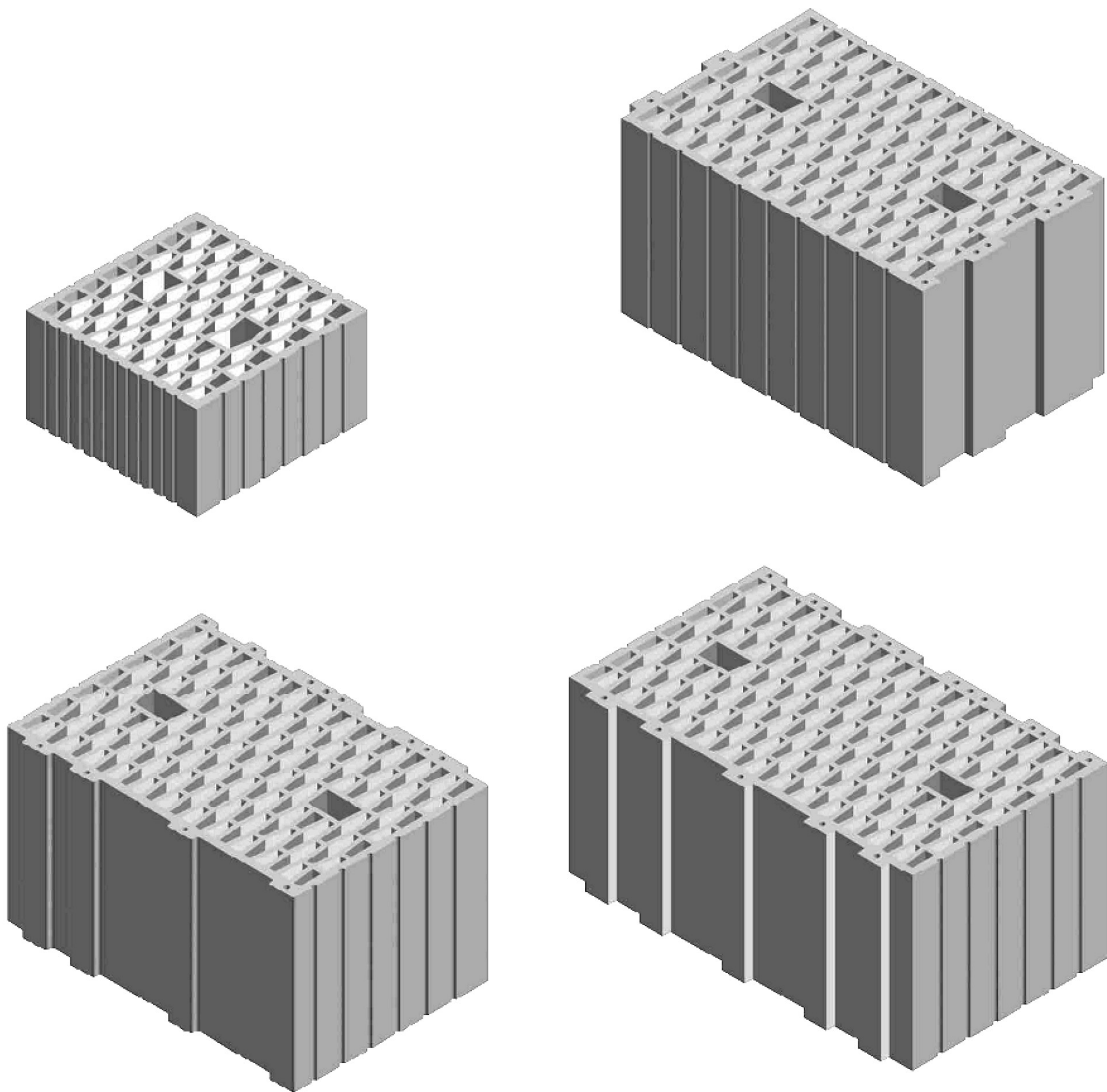
Рисунок А.4 — Камни
